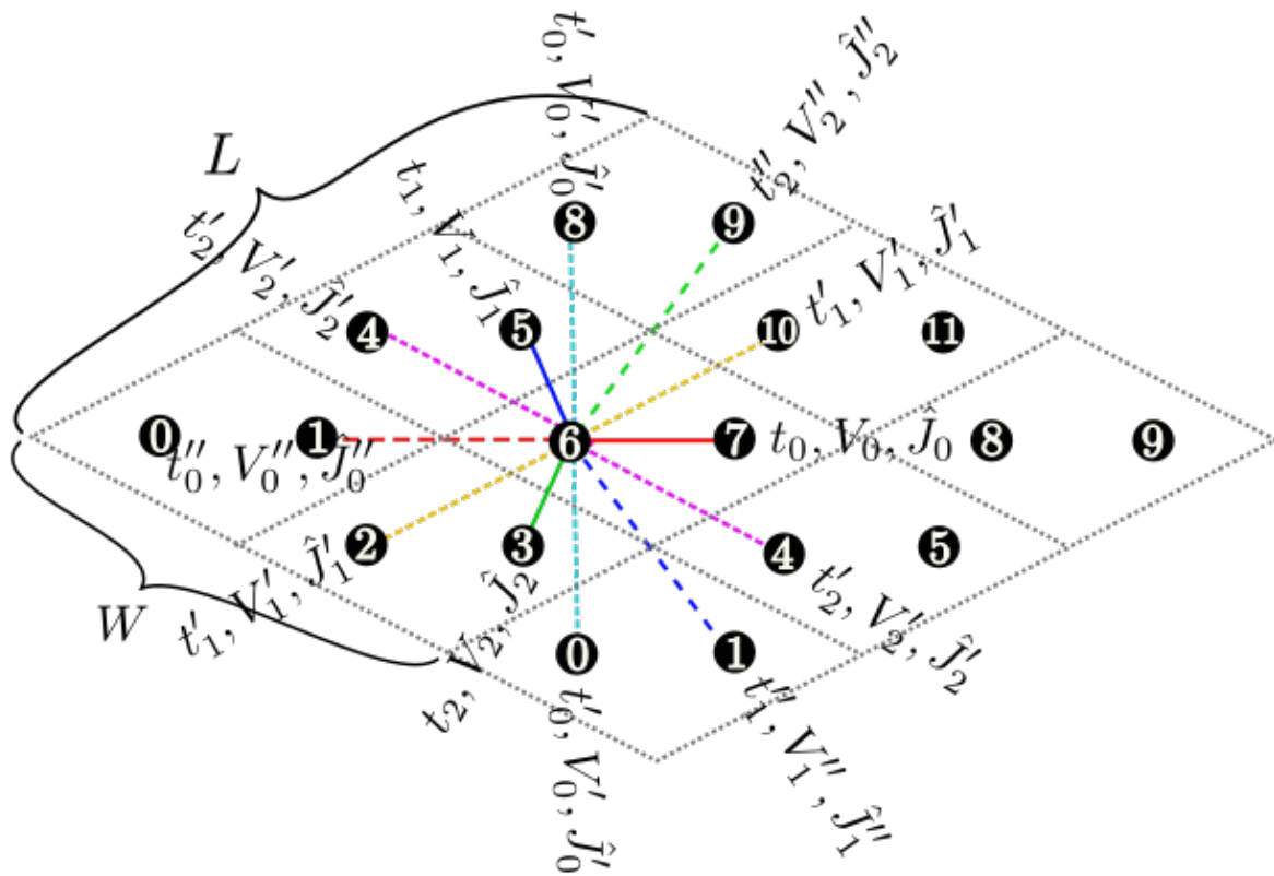
図 4.2: 2次元異方的蜂の巣格子の模式図. ホッピング積分、オフサイトクーロン積分、スピン結合は、ボンドの方向によって異なります。
