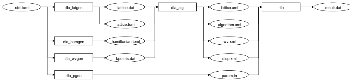
図 4.2 DSQSS/DLA のスタンダードモード. 丸囲みがファイルを, 四角囲みがツールを表す.
