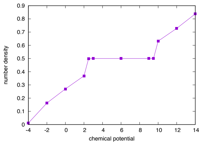
図 3.2 正方形格子上のボースハバード模型における密度の化学ポテンシャル依存性.
